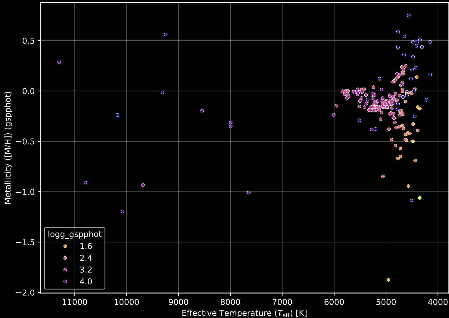
APOGEE DR17 Field: [Berkeley75] Stellar Population Parameters (n= 211)
